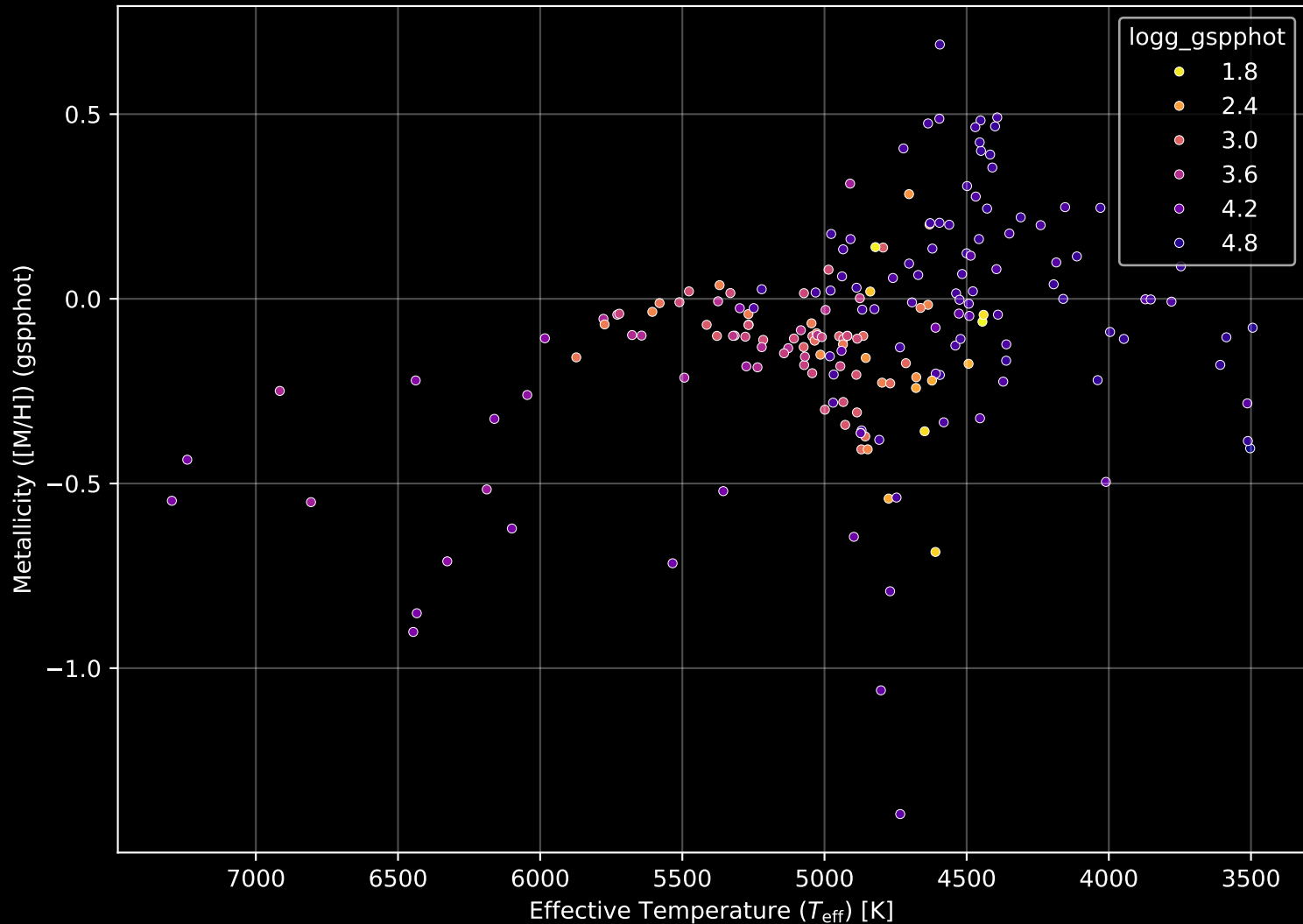
APOGEE DR17 Field: [162+34_btx] Stellar Population Parameters (n= 192)
